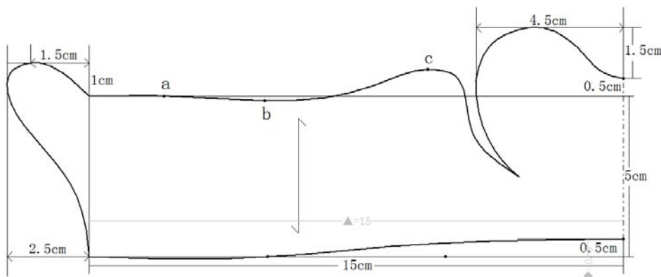
图6 虎头鞋鞋身纸样
